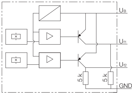
Blockschaltbild PNP
